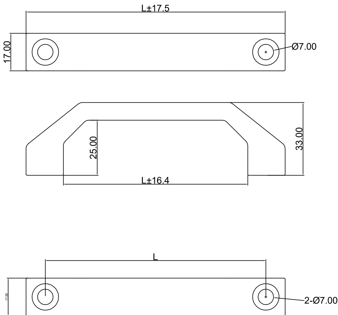
开孔尺寸
