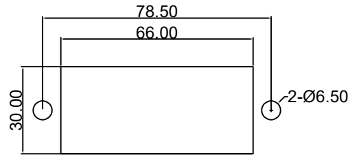
LS122-2安装孔
