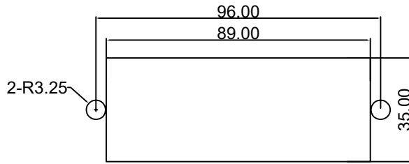
LS122-1安装孔
